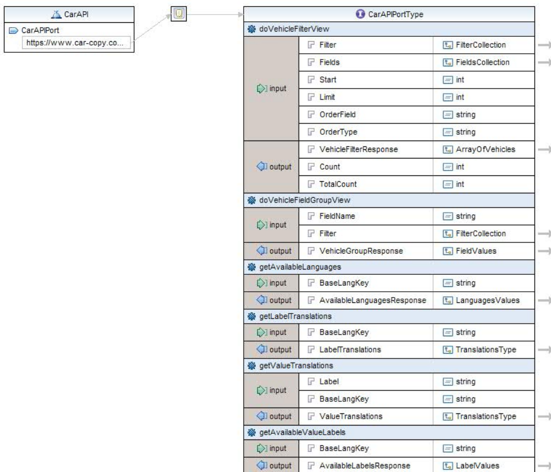
Abbildung 3.1: WSDL Schema
